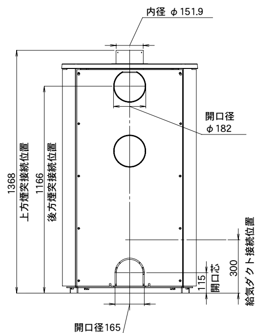
背面図
