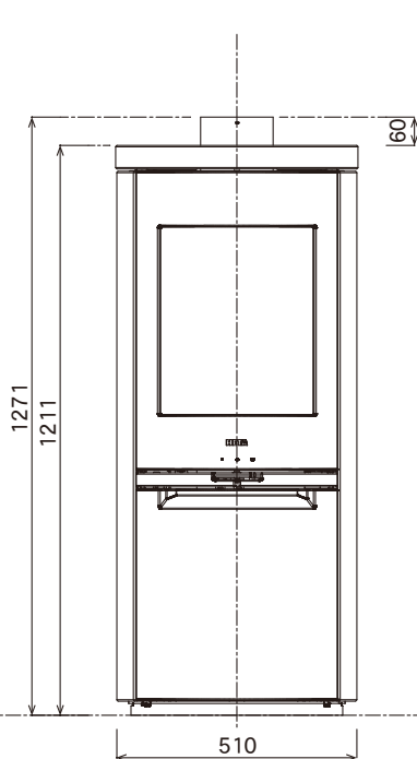
正面図
