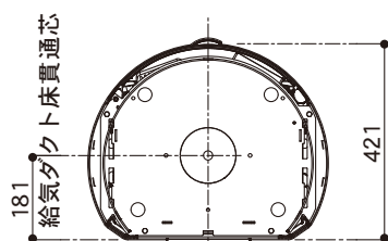
底面図
