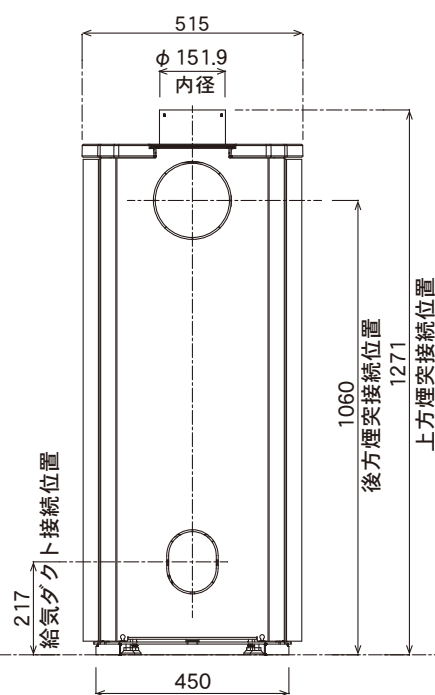
背面図
