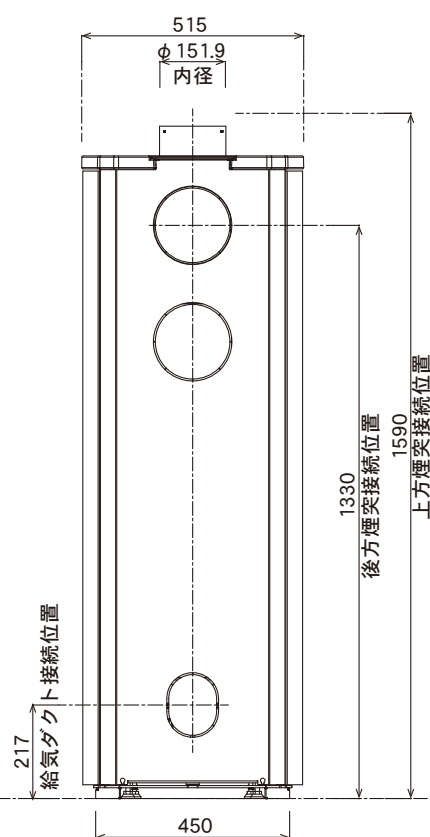
背面図
