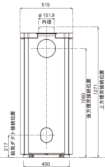
背面図
