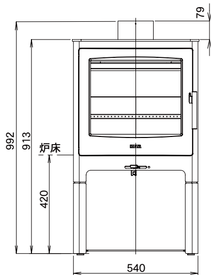
正面図
