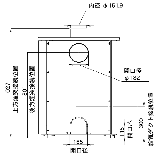
背面図
