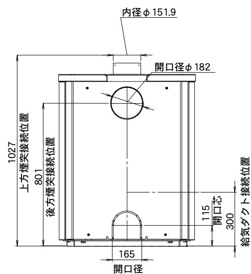
背面図
