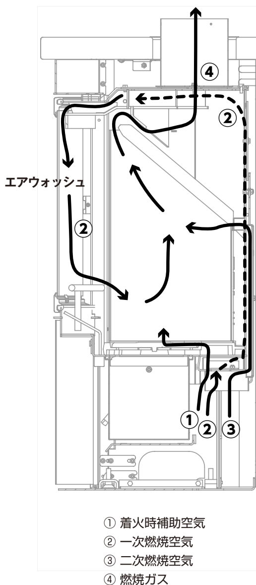
<エアフロー図>
