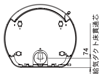
底面図
