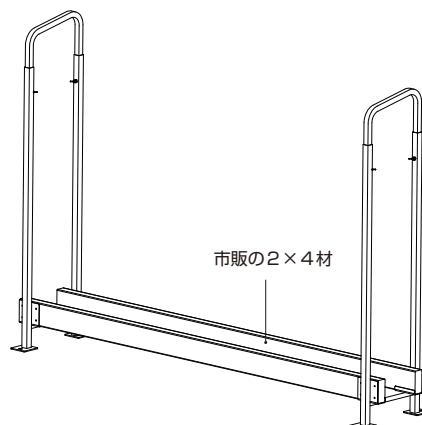
2×4ログラック スライド 30【品番：Y035】 スライド 40【品番：Y047】
