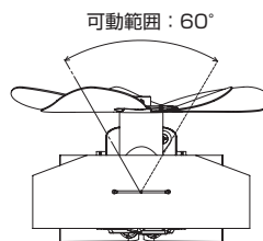
【上面図】
