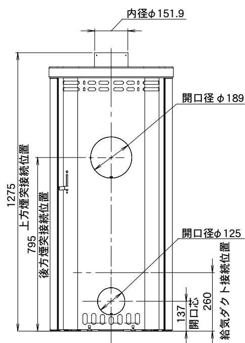
背面図
