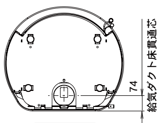
底面図
