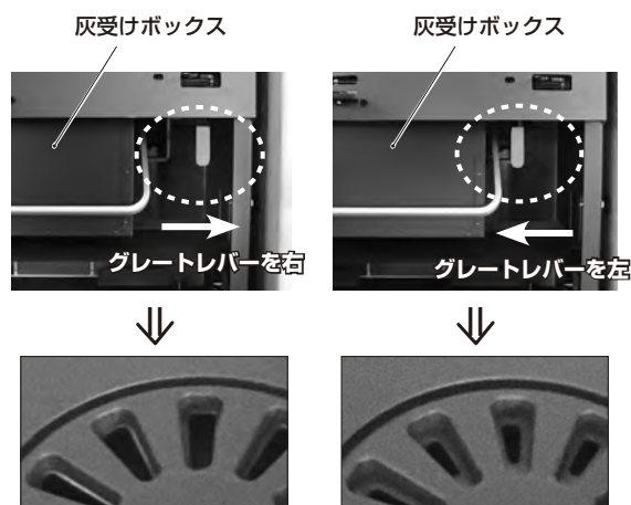
グレートレバーを右に寄せるとグレートの間隙が広くなり 左に寄せるとグレートの間隙が狭くなる
