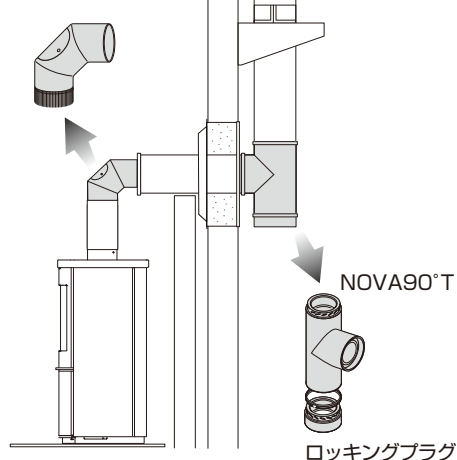
90°エルボー
