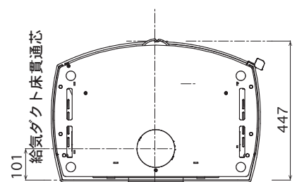
底面図
