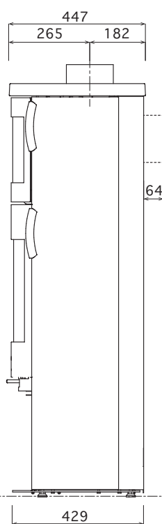
側面図
