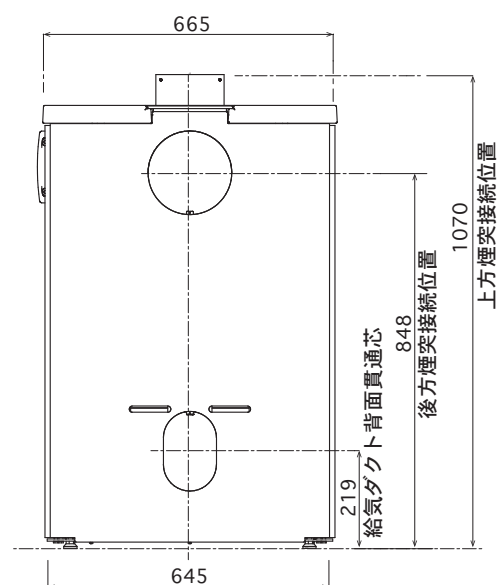
背面図
