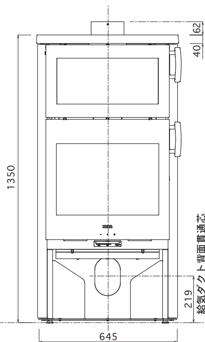
正面図
