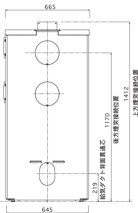
背面図
