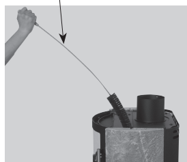
側面对流層の掃除
