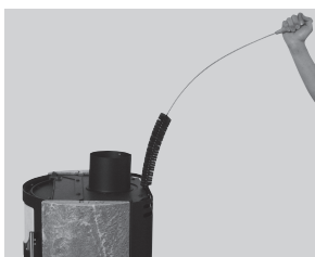
背面对流層の掃除
