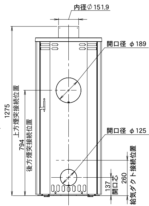
背面図
