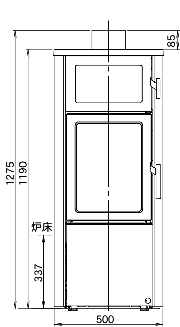
正面図
