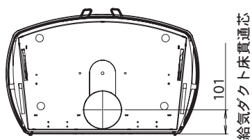
底面図
